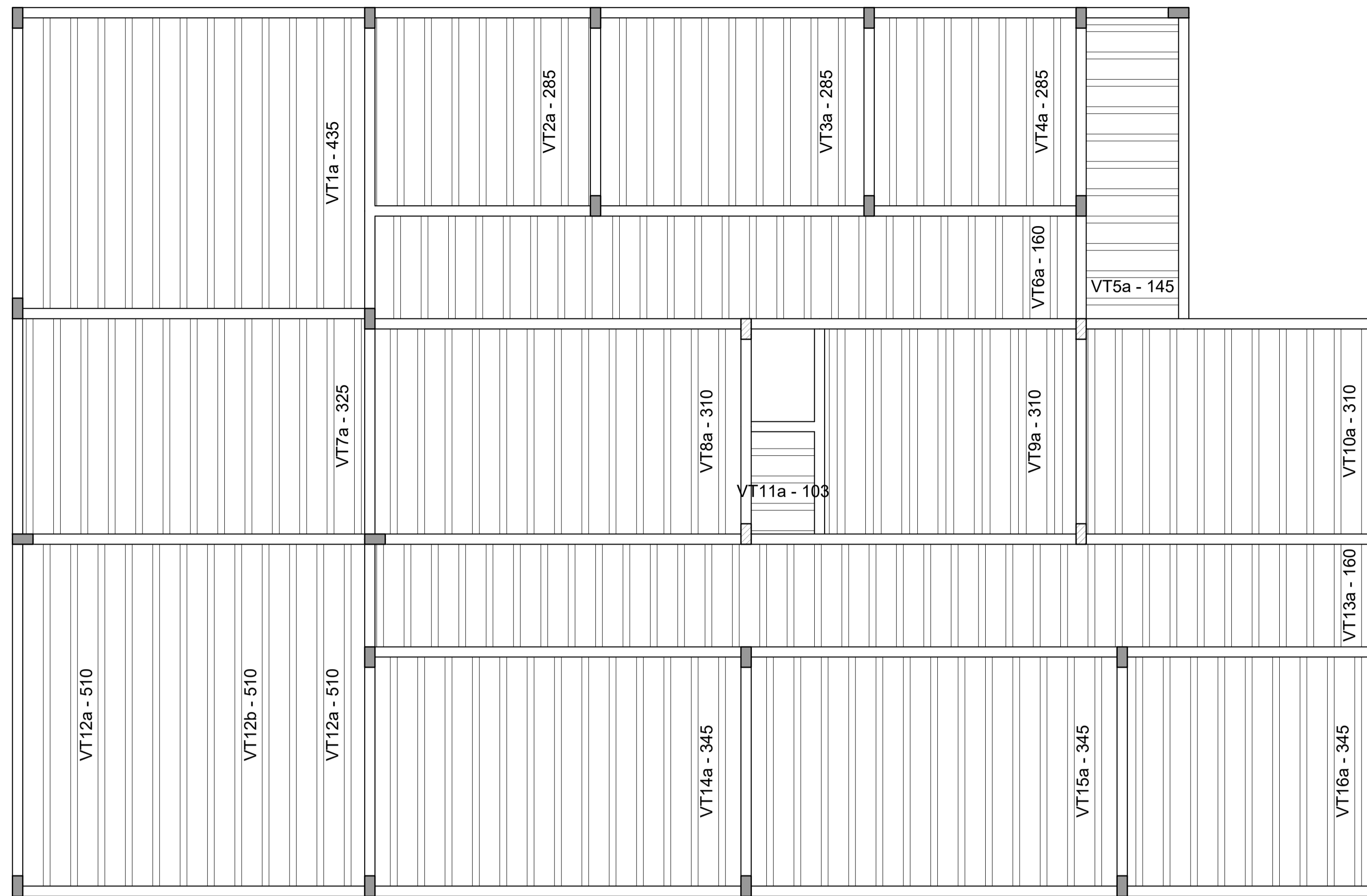
PLANTA DE VIGOTAS PRÉ-MOLDADAS Escala 1:50
